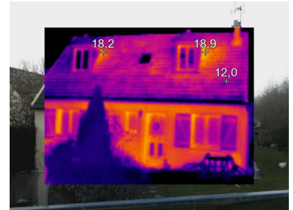
Fuite de chaleurs aux niveaux des lucarnes et des ouvrants
