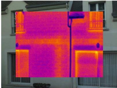
Ponts thermiques au niveau du plancher intermédiaire et du mur de refend
